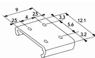
βάση στήριξης τοίχου - οροφής wall - roof support
