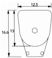
στήριξη σε οροφή roof fixing
