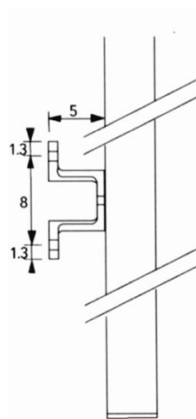
βάση στήριξης οδηγού side guide support
