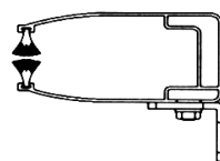
profile οδηγού 9,5cmX4,8cm side guide profile 9,5cmX4,8cm
