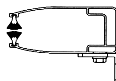
profil οδηγού 11,5cmX4,8cm side guide profile 11,5cmX4,8cm
