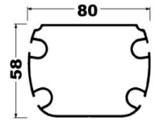
profil αντιβάρου bottom bar profile
