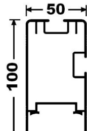
profil οδηγού / guide
